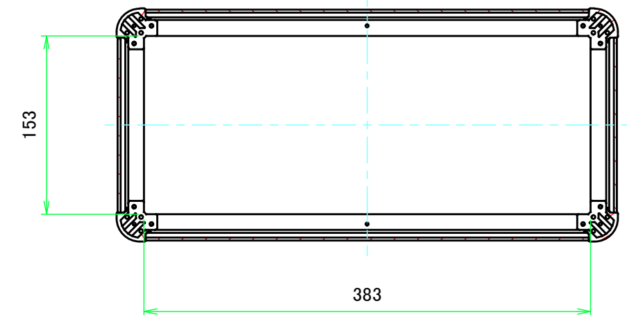
C-C (1 : 4.5)
